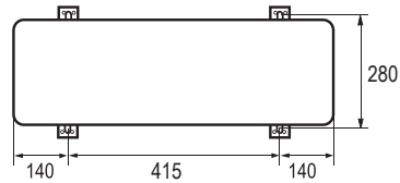
Outdoor unit floor fixing dimensions. Units in mm Algunos sistemas de 9 000 BTU/h, y algunos 12 000 BTU/h de capacidad
